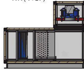
A-A (1 : 21)
